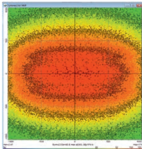
Fényeloszlás fényvisszaverővel
